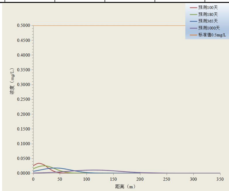
图 5.2-1 \text{NH}_3\text{-N} 地下水影响分析图
