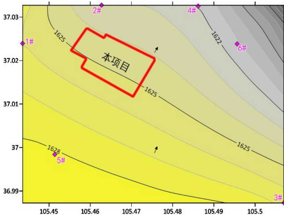
图 4.1-1 本项目所在区域等水位图
