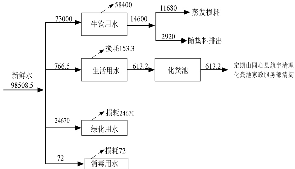
图 2.2-4 本项目水平衡图 单位 \text{m}^3/\text{a}
