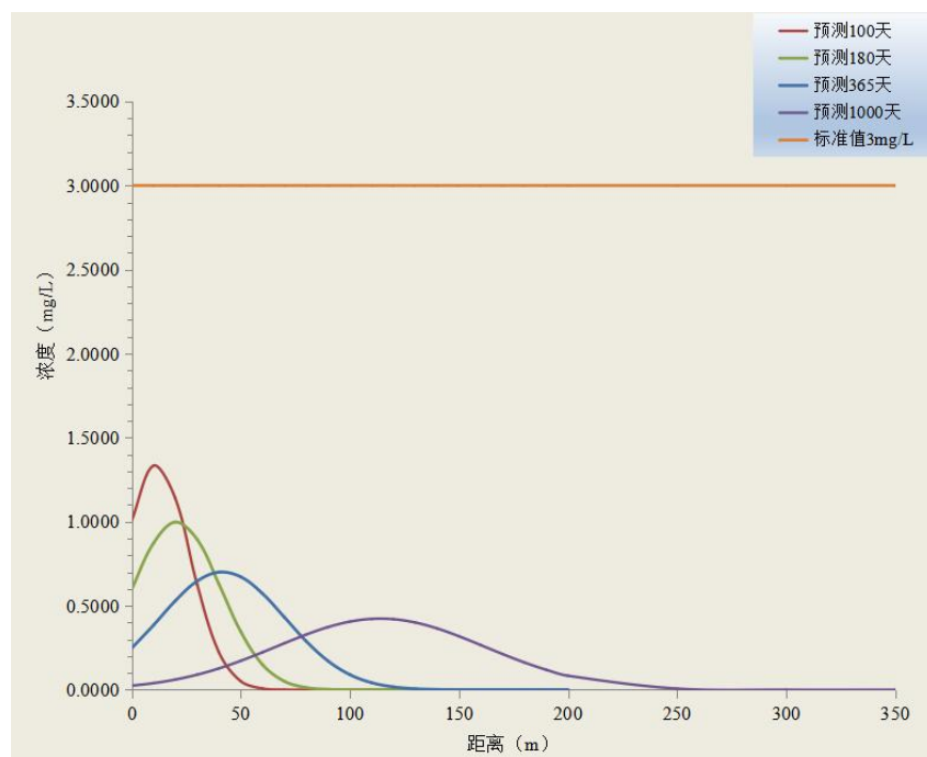
图 5.2-2 耗氧量地下水影响分析图
