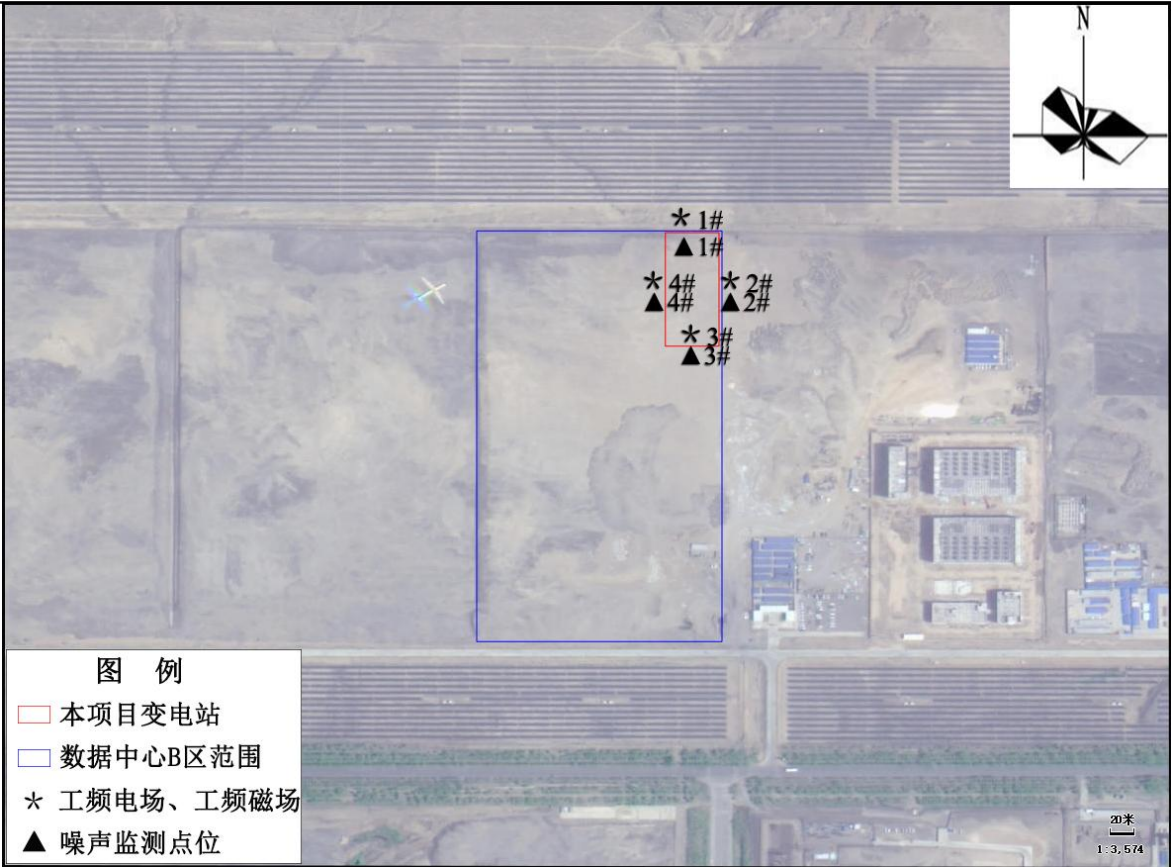
图17 电磁、噪声监测点位图
