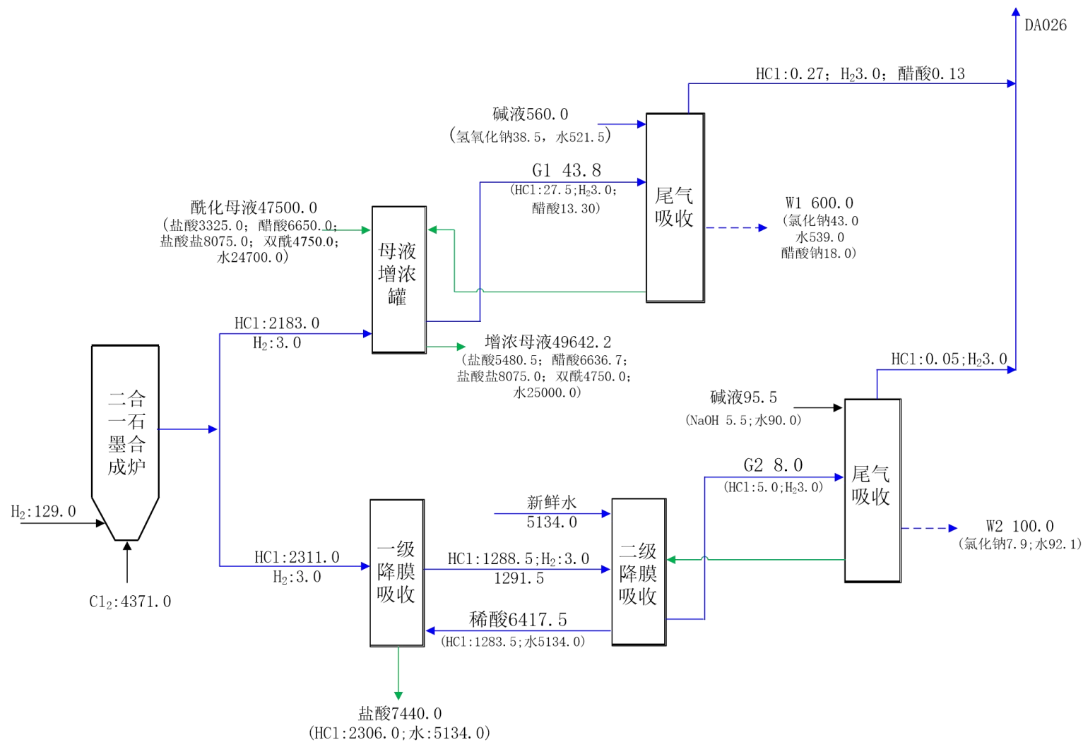
图 4.2-2 本项目物料平衡图 (t/a)
