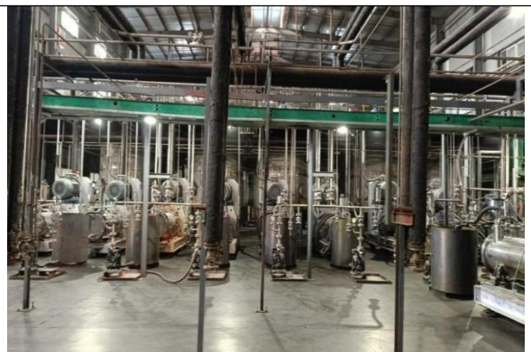
砂磨生产车间（内部）
