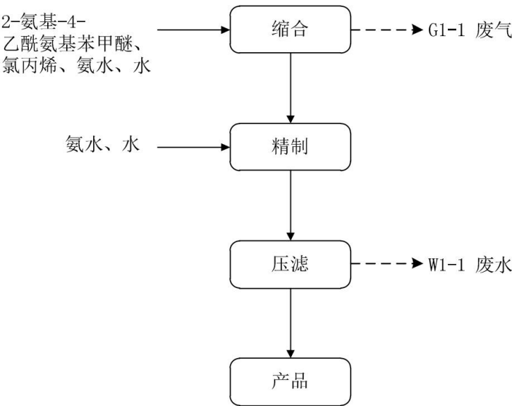
图 2.8-1 在建工程生产工艺流程图
