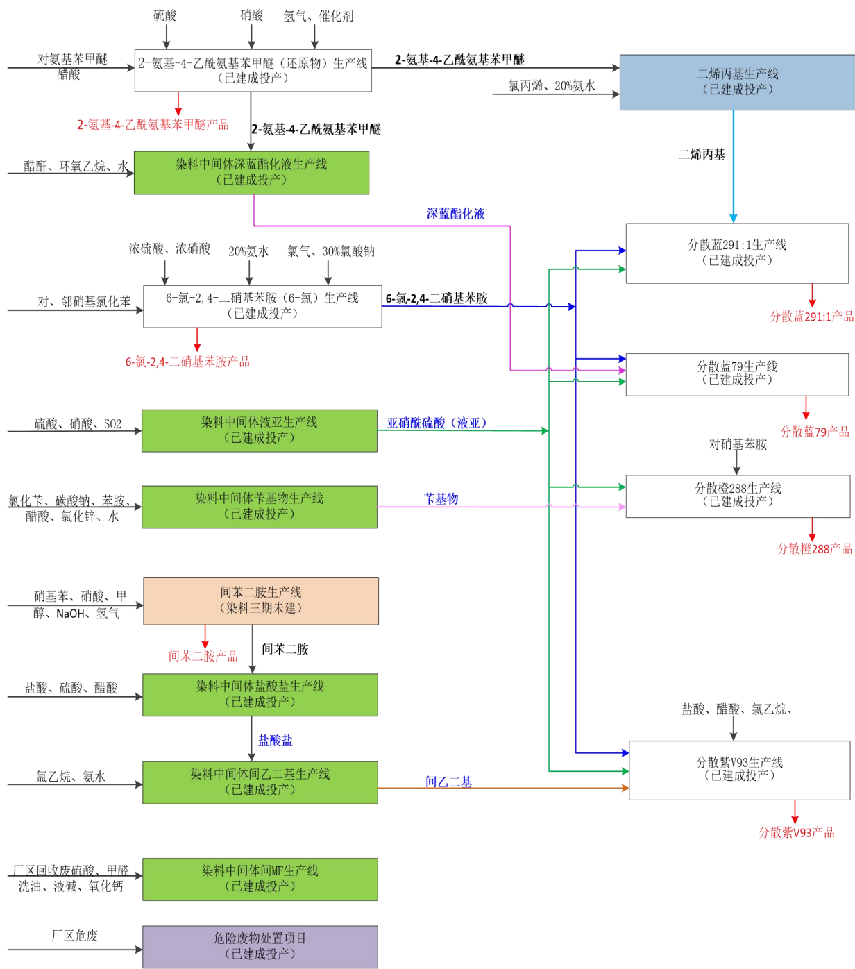
图 2.1-1 全厂产业链示意图
