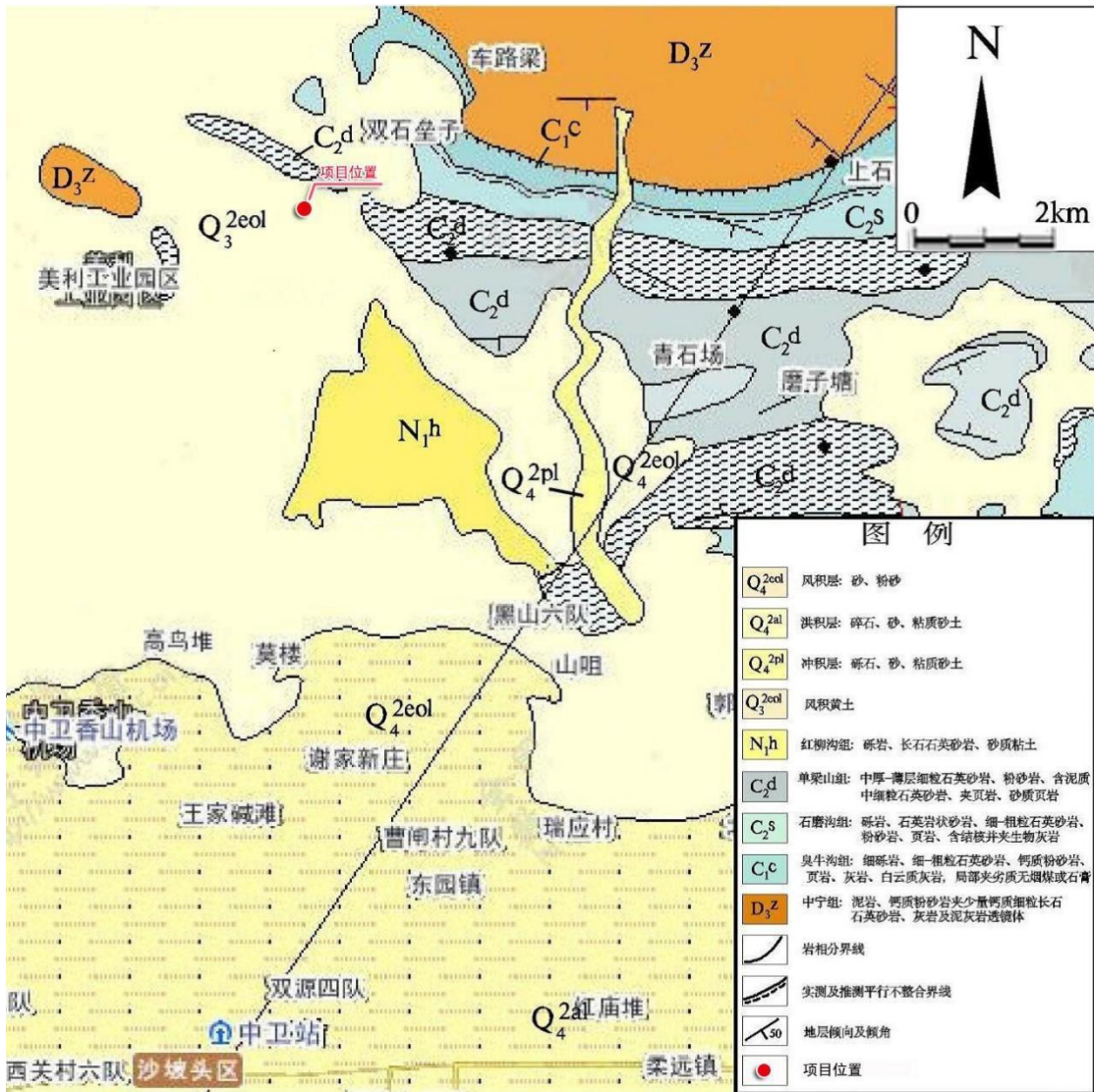
图 6.4-2 区域地质图
