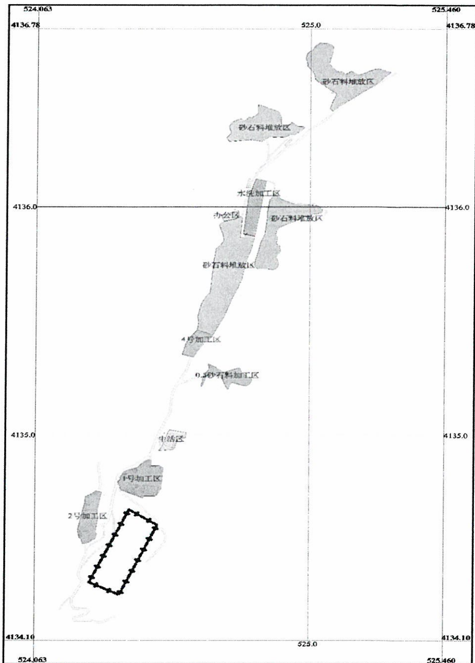
图 1-2 矿区总平面布置图
